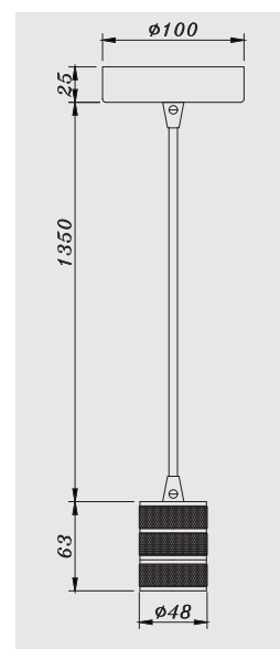
DIMENSIONS
