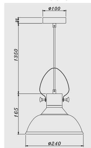
DIMENSIONS
