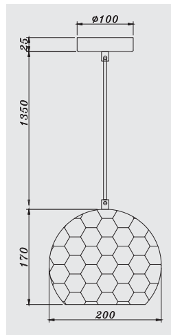
DIMENSIONS
