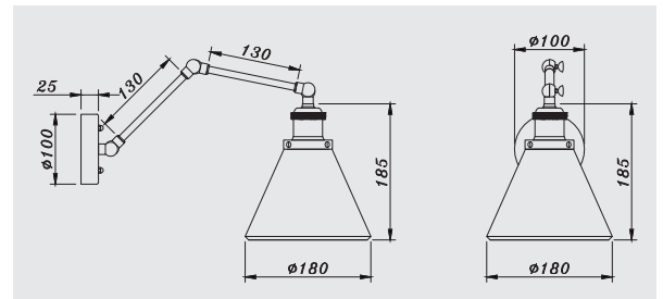
DIMENSIONS
