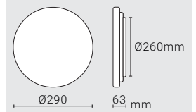
20W - DIMENSIONS
