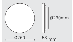
14W - DIMENSIONS
