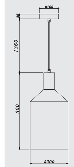
DIMENSIONS
