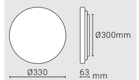
24W - DIMENSIONS
