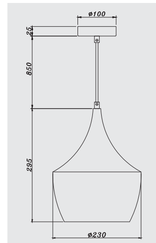
DIMENSIONS
