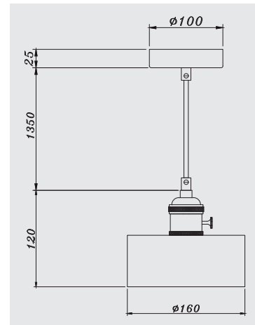
DIMENSIONS
