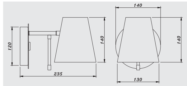
DIMENSIONS
