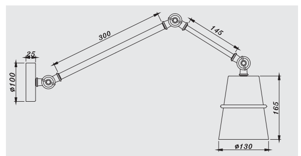
DIMENSIONS
