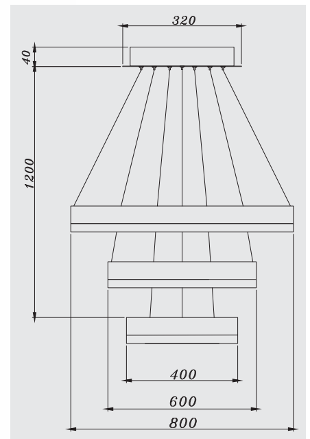
DIMENSIONS
